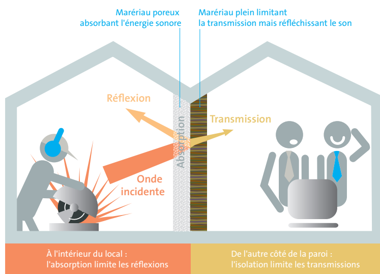
Fig. 8. Correction acoustique. Ne pas confondre correction acoustique en absorption et isolation acoustique
